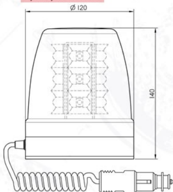
Wymiary LBL-20K1N
