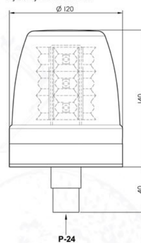
Wymiary LBL-20K1DIN
