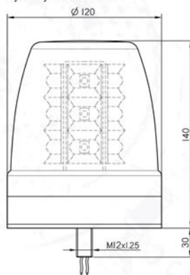
Wymiary LBL-20K1K
